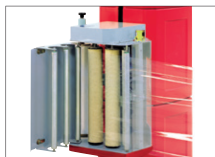
Für Maschinen mit zwei Dehnwalzen
